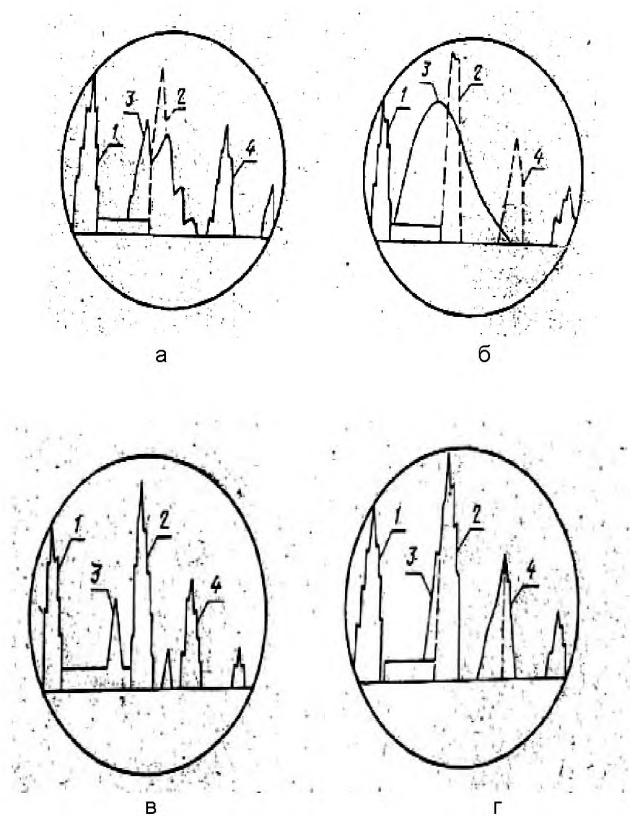
Рисунок В.1— Вид эхо-сигналов на экране дефектоскопа
